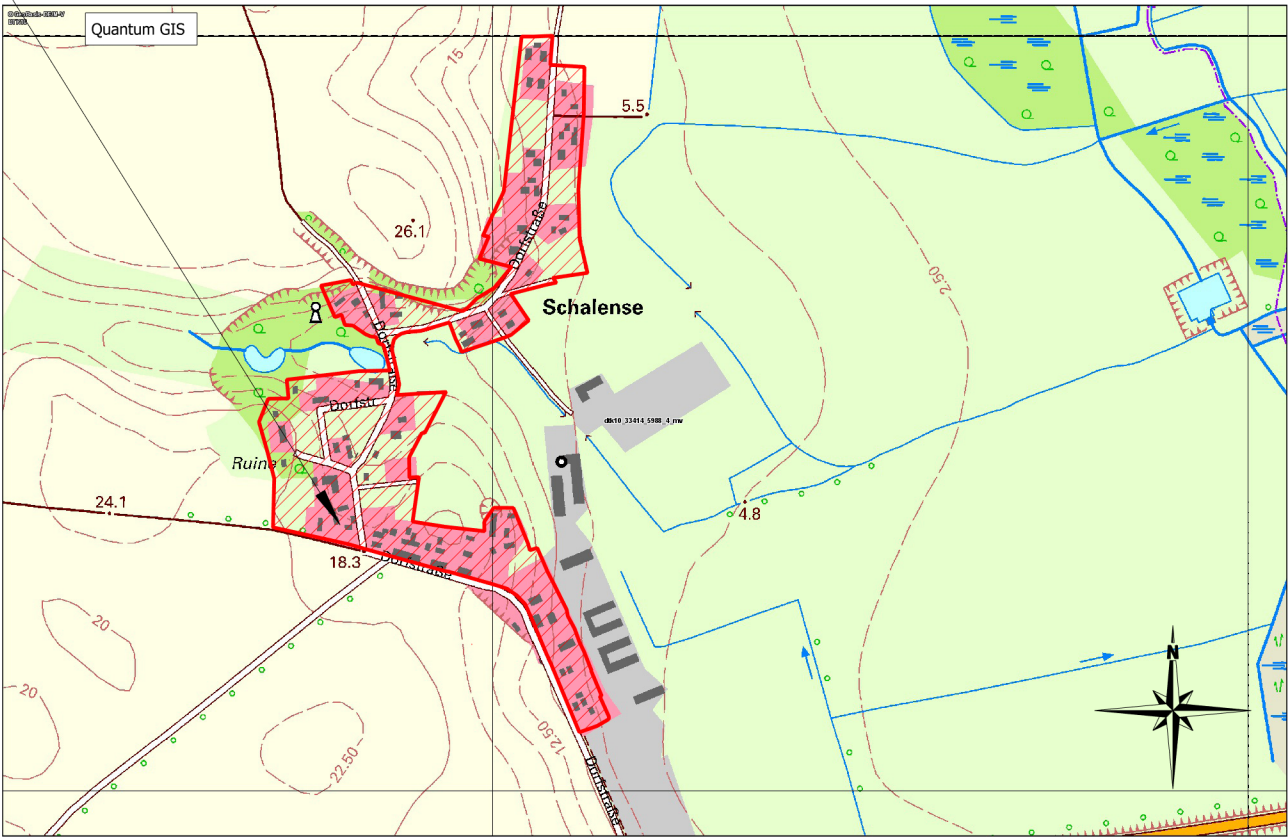
Übersichtsplan M 1 : 10.000
